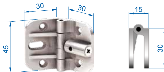
пружинная петля, серебро монтаж только в плоскости дверного полотна
